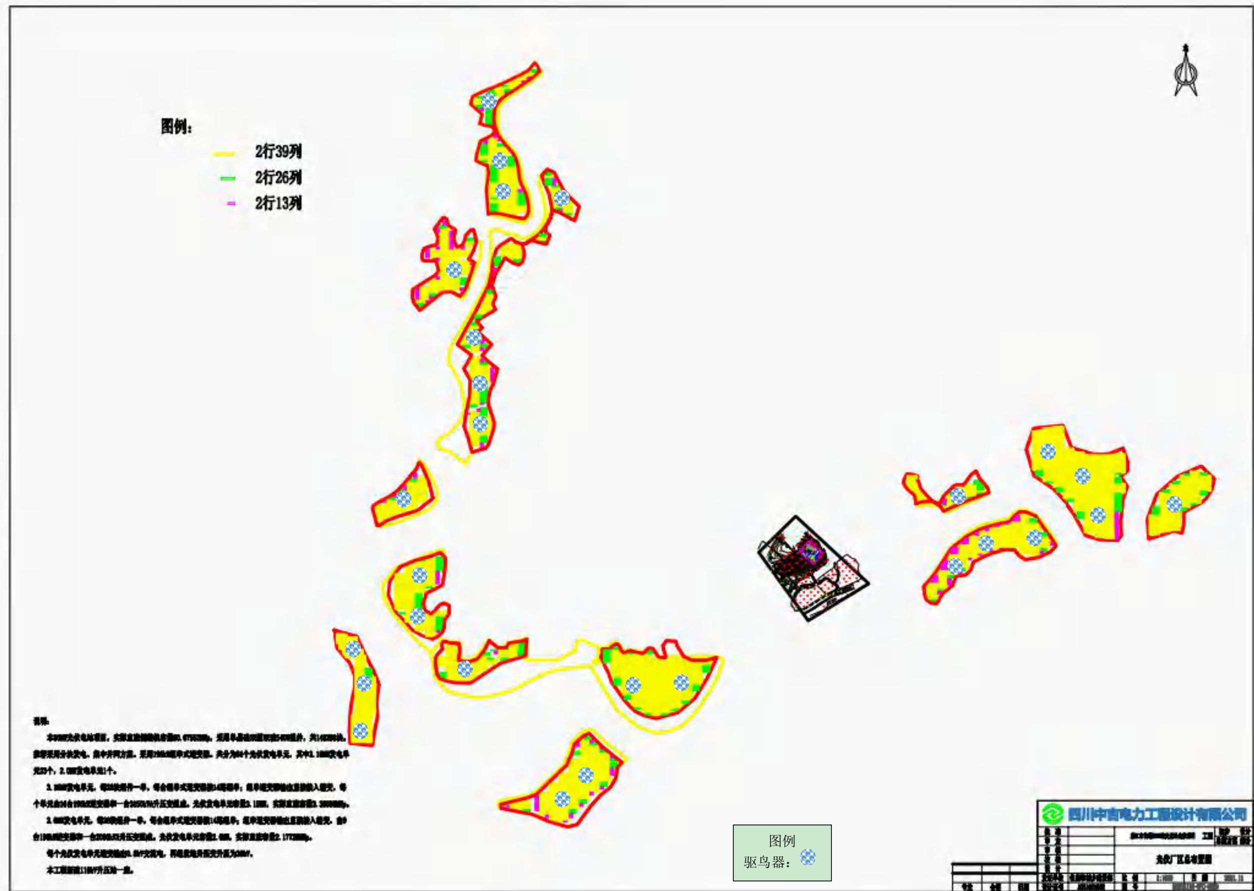
附图5 项目光伏区平面布置及生态环境保护措施分布图
