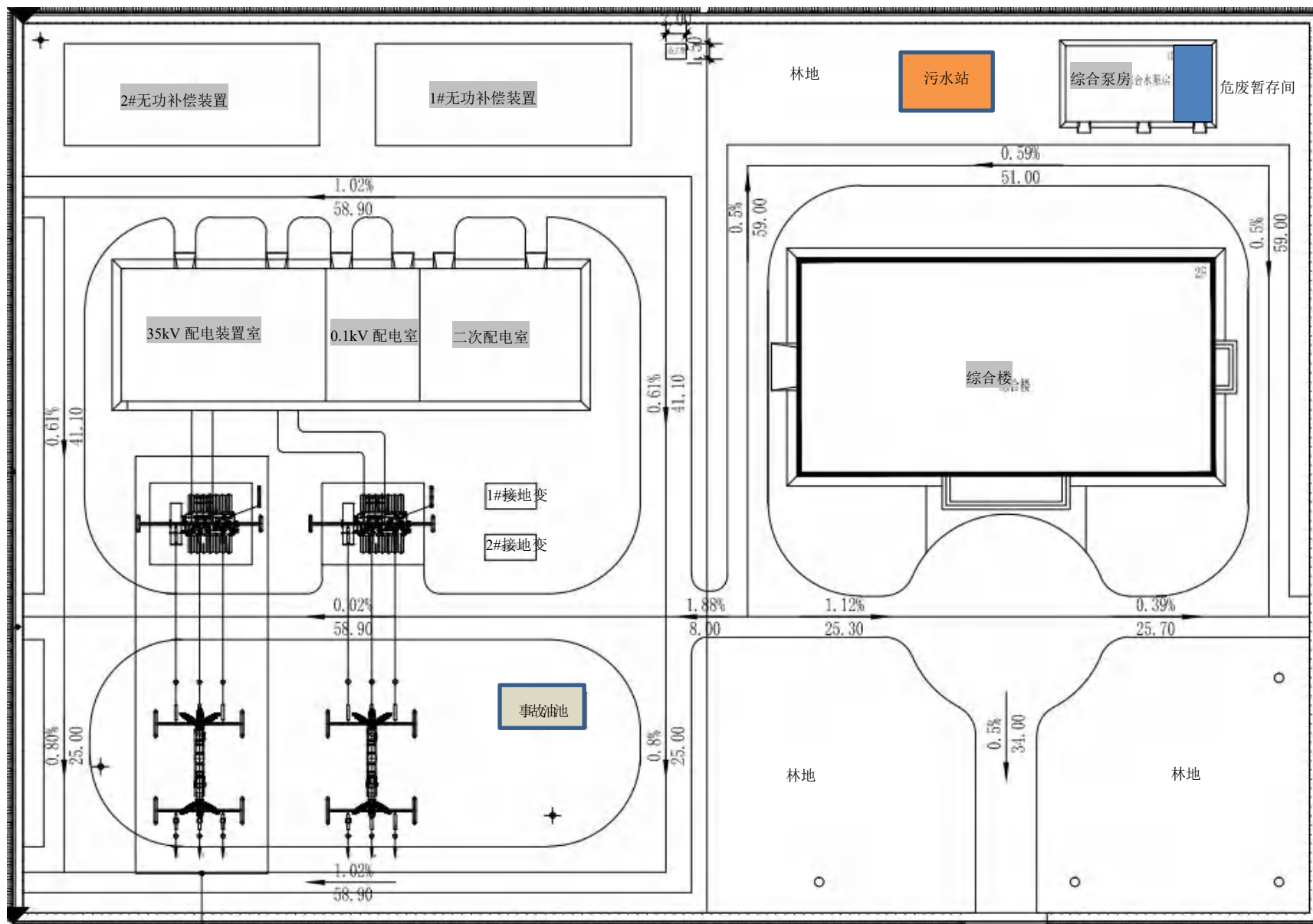
附图6 项目升压站平面布置图
