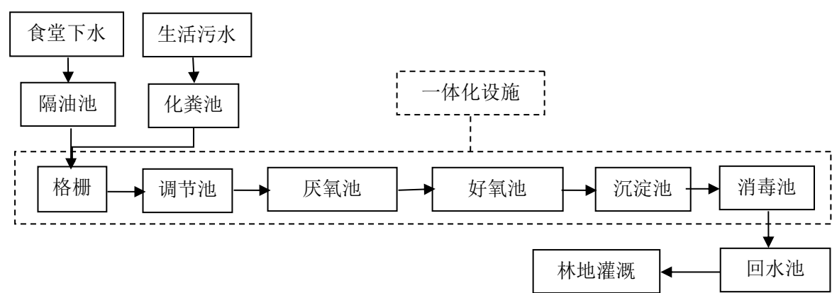
图 5-1 埋式一体化生活污水处理工艺流程图
