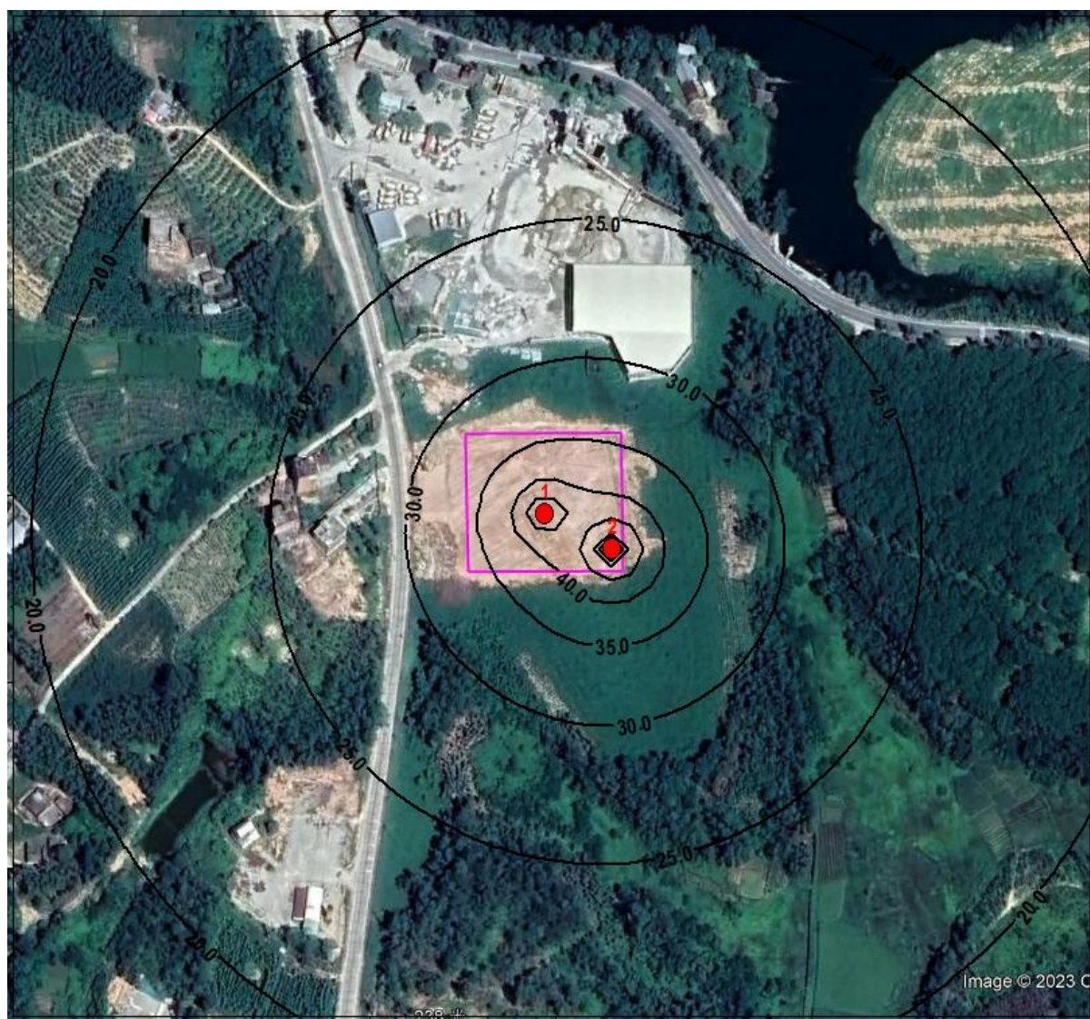
图 4-2 项目噪声贡献值等声值线图
