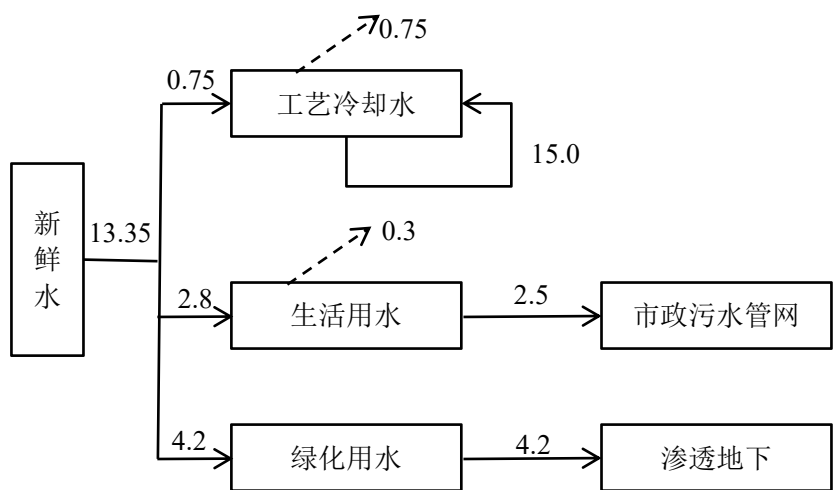
图 2-2 项目水平衡图（单位：t/d）
