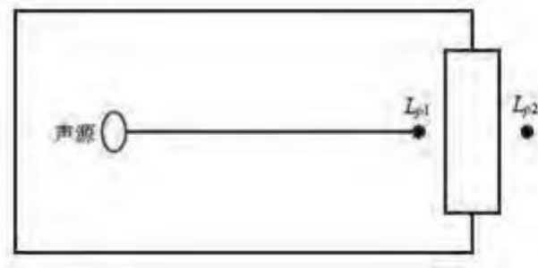
图 4-6 室内声源等效为室外声源图例
