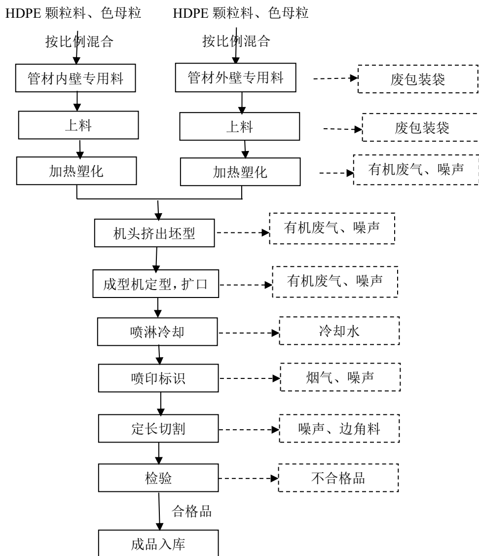
图 2-3 HDPE 双壁波纹管生产工艺流程图
