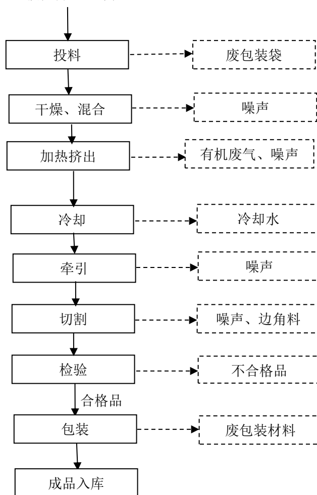
图 2-5 MPP 牵引管生产工艺流程图
