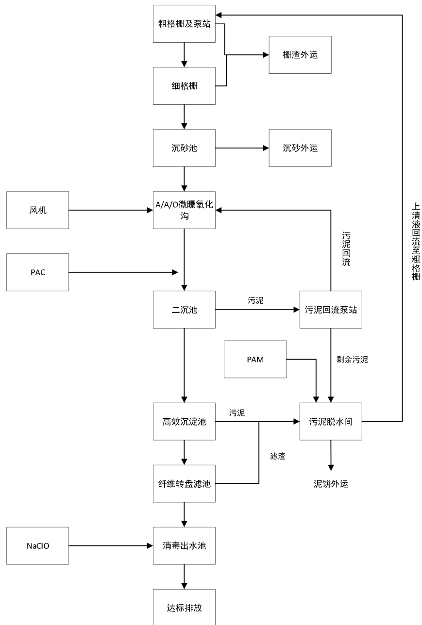
图 4-3 雷州市污水厂污水处理工艺流程图
