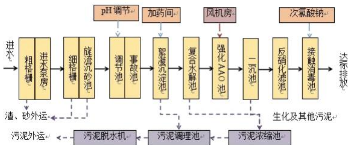
图 4-1 园区污水处理工艺流程图
