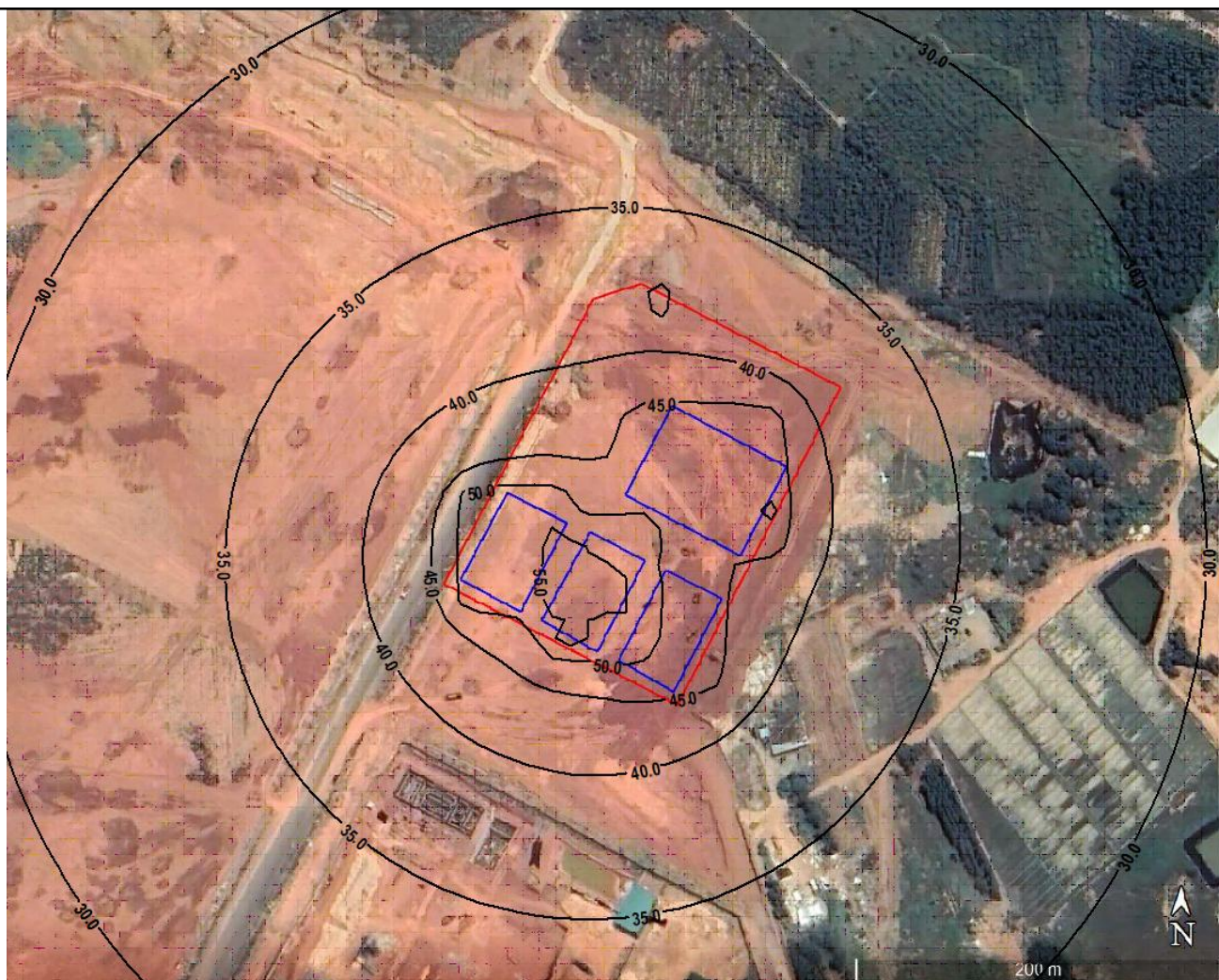
图 4-7 项目噪声贡献值等声值线图
