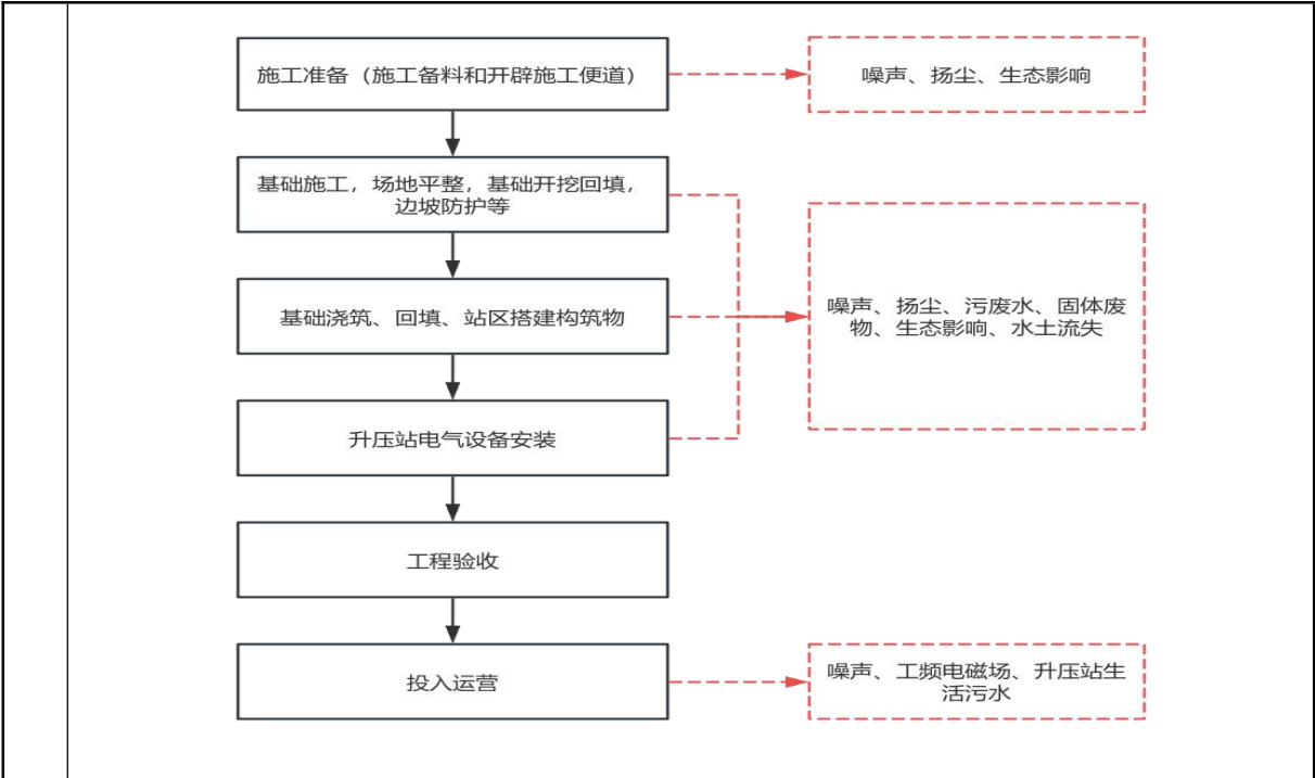
图 2-1 本工程施工期工艺流程图
