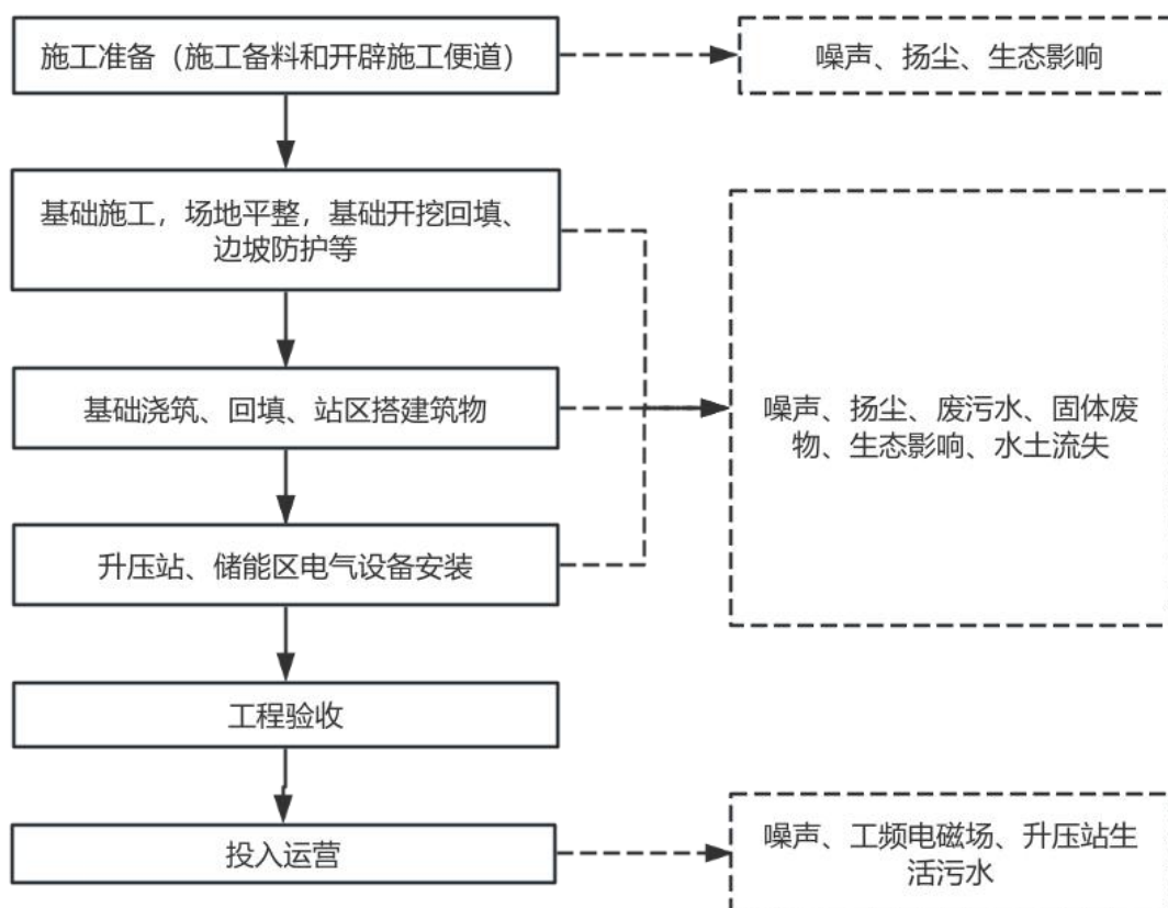
图 4-1 本工程施工期工艺流程及产污位置图
